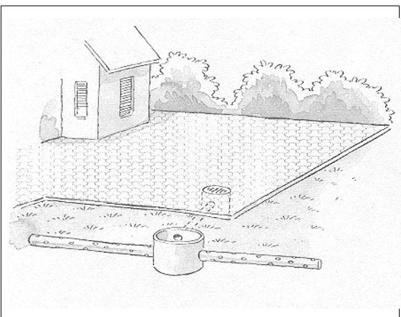
4) Versickerungs-Strang / -Galerie
